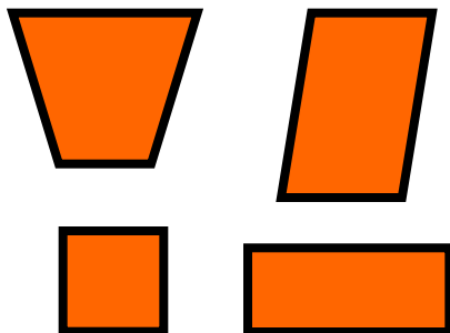
quadrilateral
