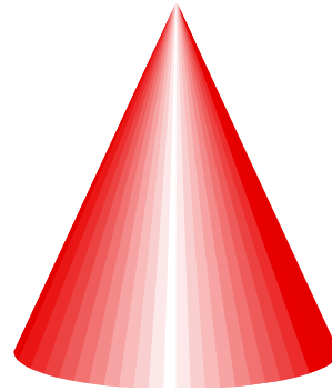
cone
