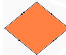
rhombus
