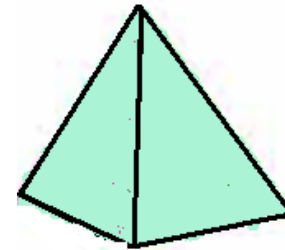
pyramid
