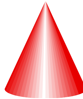
cone
