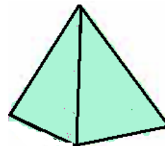
pyramid
