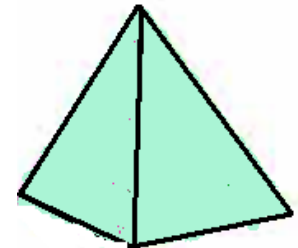
pyramid
