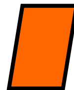
quadrilateral
