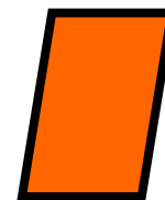
quadrilateral
