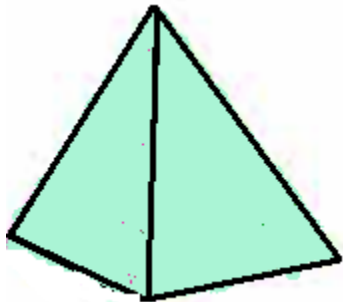
pyramid
