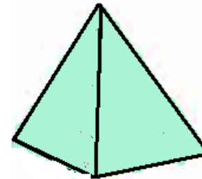
pyramid
