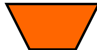
trapezium
