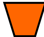
quadrilateral
